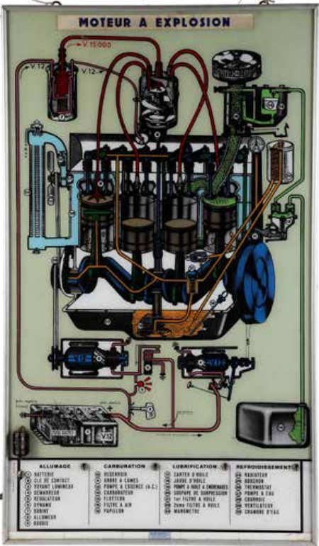
388 ECOLAUTO Tableau pédagogique lumineux montrant le fonctionnement du moteur à explosion, fonctionnel Ecolauto SA 110 x 64 x 11 cm env.
