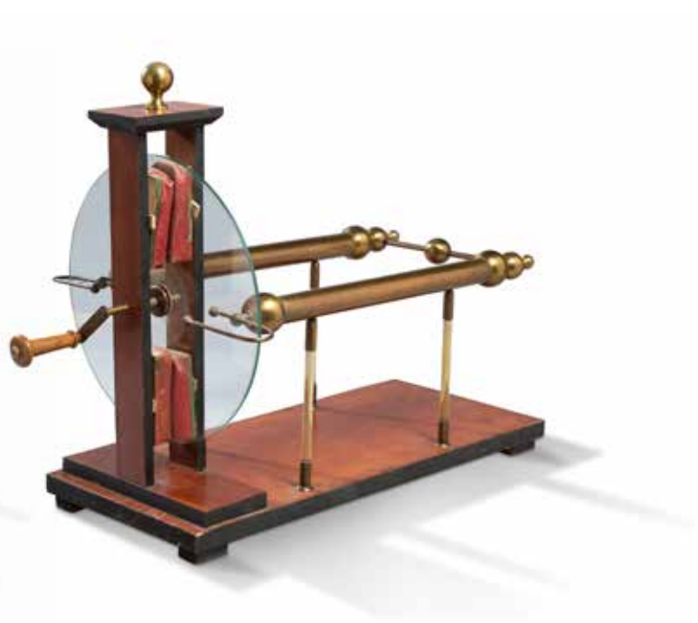
89 Machine électrostatique de Ramsden En métal, laiton et verre sur socle en bois H. 44 x L. 57 x P. 29 cm
