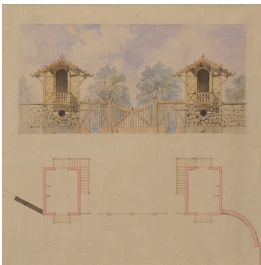
44. Pavillon de jardin. Crayon. 21 x 19,5 cm.
