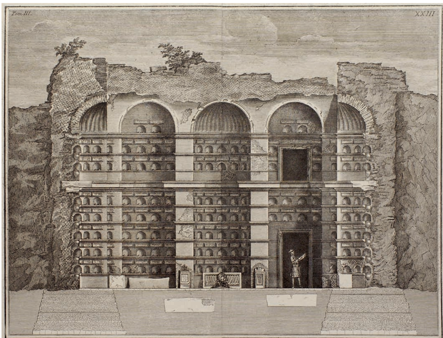
ALTRO SPACCATO della CAMERA SEPOLCRALE de' LIBERTI e SERVI della Famiglia di AVUGUSTO. Questa Parte, che forma un fianco della Camera corrispondente in tutto al fianco opposto è divisa in tre Nichioni di eguale larghezza. Quel di mezzo fatto a semicircolo ha la volta ornata similmente di stucco a figura di conchiglia. Gli altri due sono quadrati, in un de quali dal lato sinistro si veggono le due Porte, che daranno l'ingresso nella Stanza: l'una al piano l'altra sopra il Conoscimento. In tutti e tre con profila sinistra sono distribuiti gli ordini de' Colombi, come nella Parte di faccia già dimostrata. Entrando per la Porta del piano si vede al primo Pilastro un Cippo fidebre di marmo statuario colla sua Inscrizione. Al Nichione di mezzo un Avello parimente di marmo scolpito di varie marcherie scortiche con molti altri consimili ornamenti. Nell'altro che segue, si trova un Sarcofago di creta cotta. È stato osservato, che dentro lo stesso in un canto eravi un certo rialzo pur di terra cotta perugiata, alto e largo non più di once sei, il quale pare, che dovesse servire come di guanciale al defunto.
